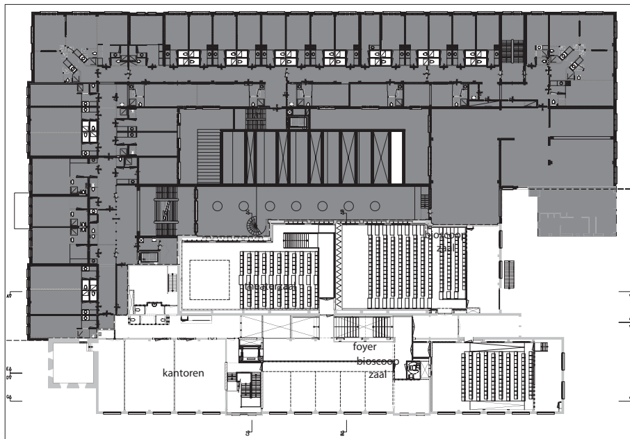
1 e verdieping
